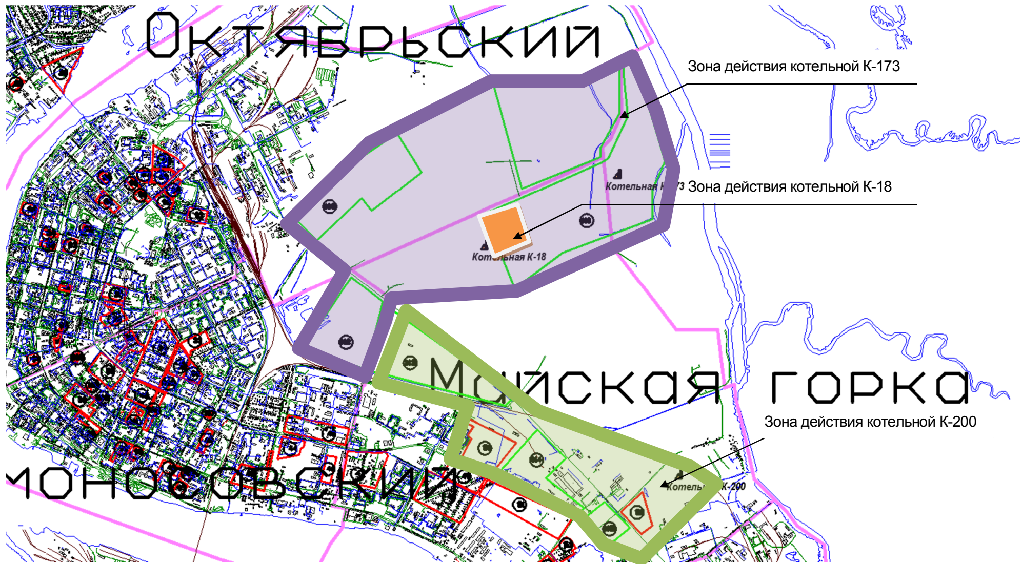
Рисунок 3.1. Предлагаемые зоны деятельности в зонах обслуживания предлагаемых к строительству котельных К-200, К-173, К-18
